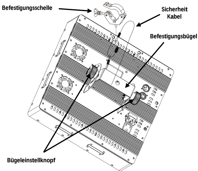
Montageansicht
