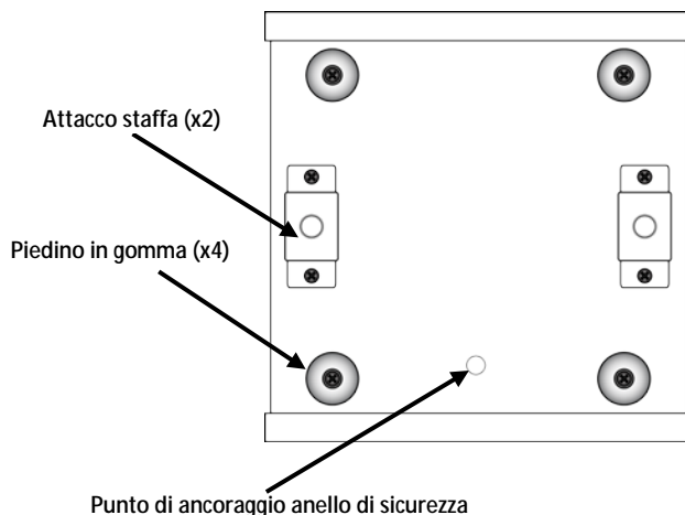
Schema di Montaggio Dell'unità
