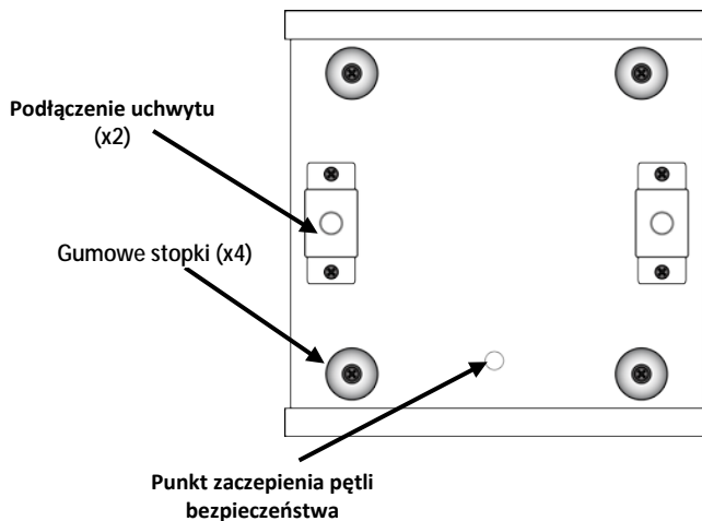
Rysunek Montażu Produktu
